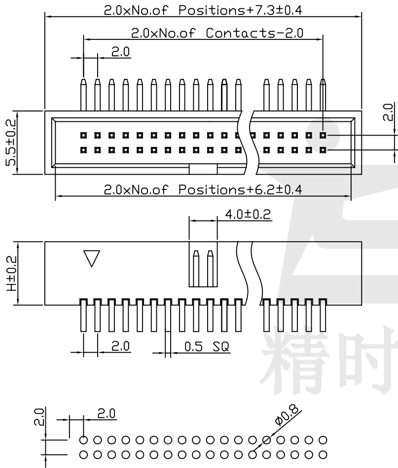
P.C.B LAYOUT
