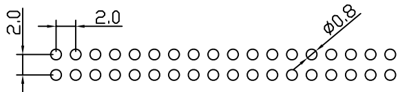
P.C.B LAYOUT
