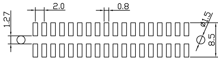
P.C.B LAYOUT
