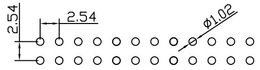
P.C.B LAYOUT
