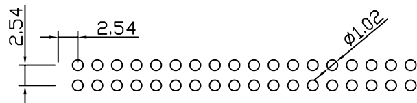
P.C.B LAYOUT
