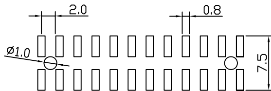
P.C.B LAYOUT
