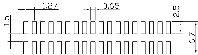
P.C.B LAYOUT
