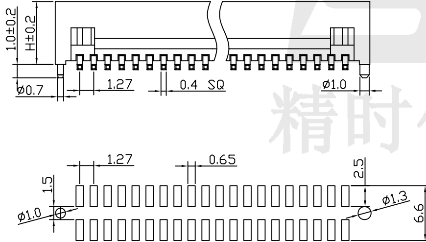
P.C.B LAYOUT
