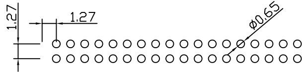
P.C.B LAYOUT
