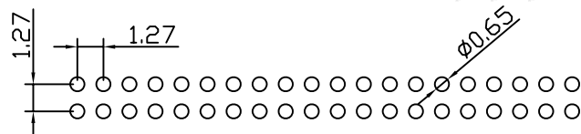
P.C.B LAYOUT
